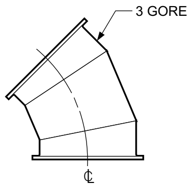
45° ELBOW
