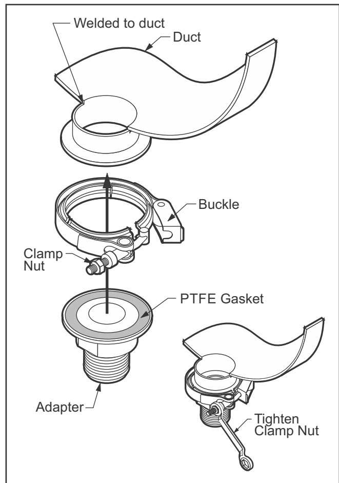
Fig. 50: Fab-Tech Flange Assembly
